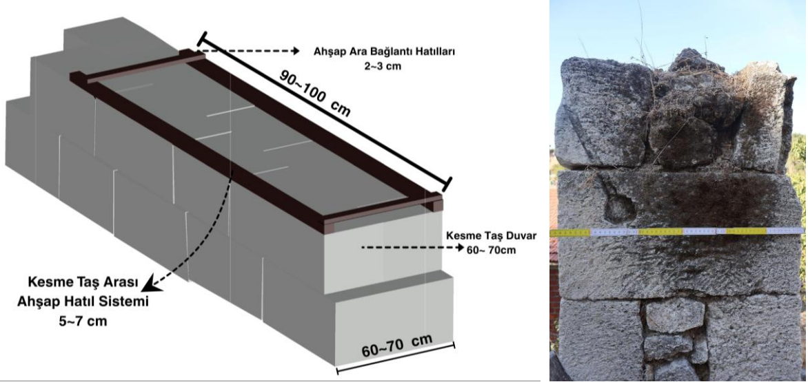
Şekil 15. Misvak Köyü'nde Gözlemlenen Taş Duvarların Ahşap Hatıl ile Birleşim Detayları ve Taş Duvar Kesiti, Eylül 2025.
